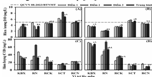
Hình 4. Diễn biến hàm lượng DO (A, B) và COD (C, D) ở 2 đợt tại 5 tuyến kênh khảo sát Ghi chú: Như hình 3.
