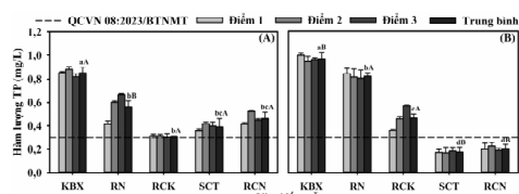
Hình 6. Diễn biến hàm lượng TP (A, B) ở 2 đợt tại 5 tuyến kênh khảo sát
