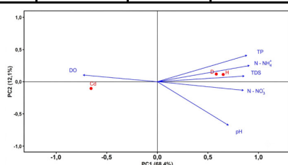
Hình 8. Biểu đồ phân tích PCA mối liên hệ giữa chất lượng nước và ĐDSH
