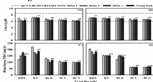
Hình 3. Diễn biến giá trị pH (A, B) và hàm lượng TDS (C, D) ở 2 đợt tại 5 tuyến kênh khảo sát
