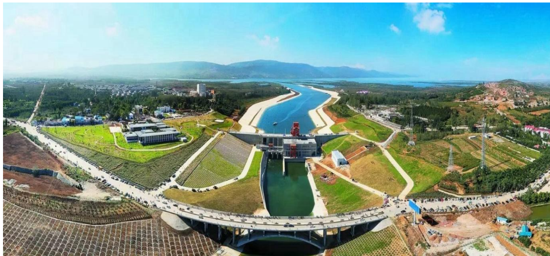
Hình 1. Điểm đầu của tuyến chuyển nước phía Đông (Trung Quốc)
