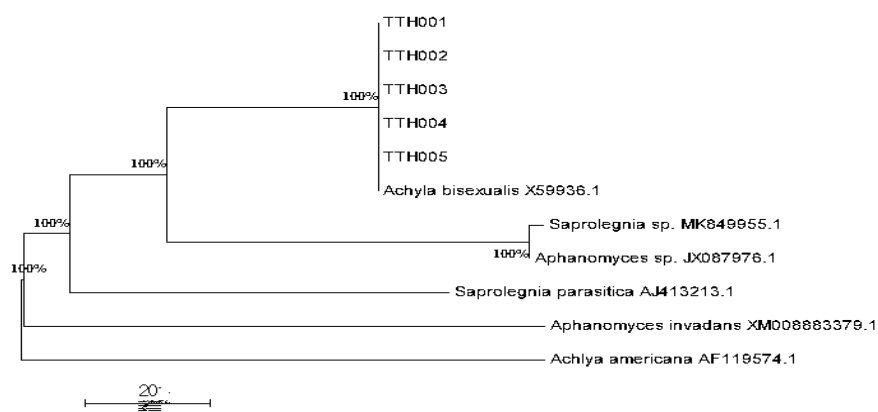
Hình 4. Cây phả hệ của 5 chủng nấm phân lập trên cá tằm với mô hình Tamurai-Nei thực hiện trên phần mềm MEGA 6.0
