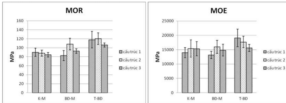
Hình 3. Độ bền uốn tĩnh (MOR) và mô đun đàn hồi khi uốn tĩnh (MOE) ván LVL với các cấu trúc xếp lớp khác nhau
