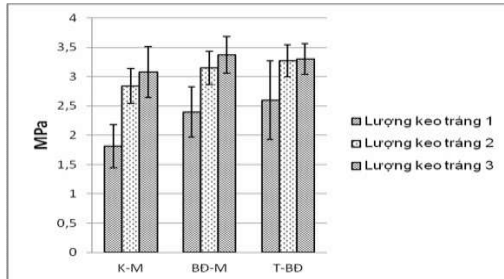
Hình 4. Độ bền dán dính ván LVL với các lượng keo trắng khác nhau
