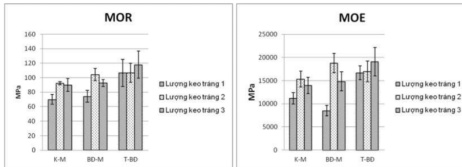
Hình 5. Độ bền uốn tĩnh (MOR) và mô đun đàn hồi khi uốn tĩnh (MOE) ván LVL với các lượng keo trắng khác nhau
