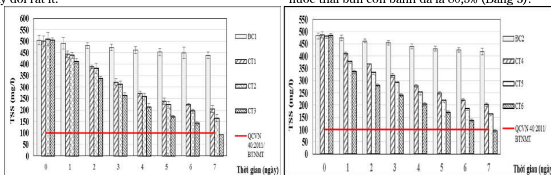
Hình 2. TSS nước thải qua các ngày
