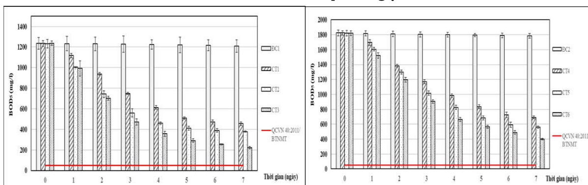
Hình 4. BOD 5 nước thải qua các ngày
