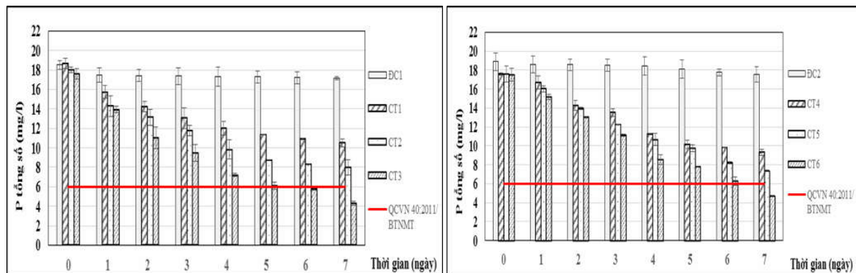
Hình 6. Photpho tổng số nước thải qua các ngày
