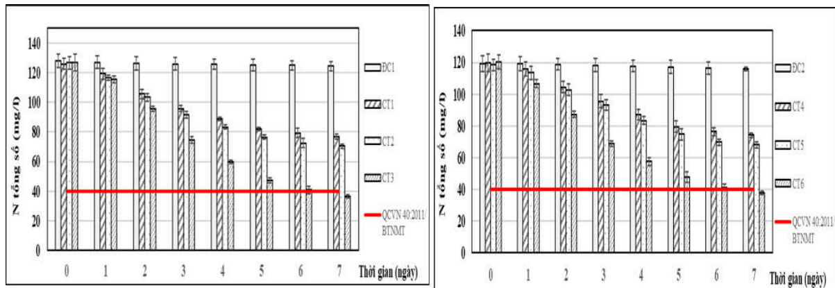
Hình 5. Nitơ tổng số nước thải qua các ngày
