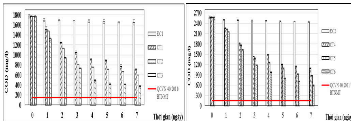
Hình 3. COD nước thải qua các ngày
