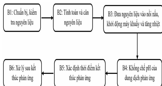
Hình 1. Sơ đồ quy trình công nghệ sơ bộ sản xuất keo UF - KC113
