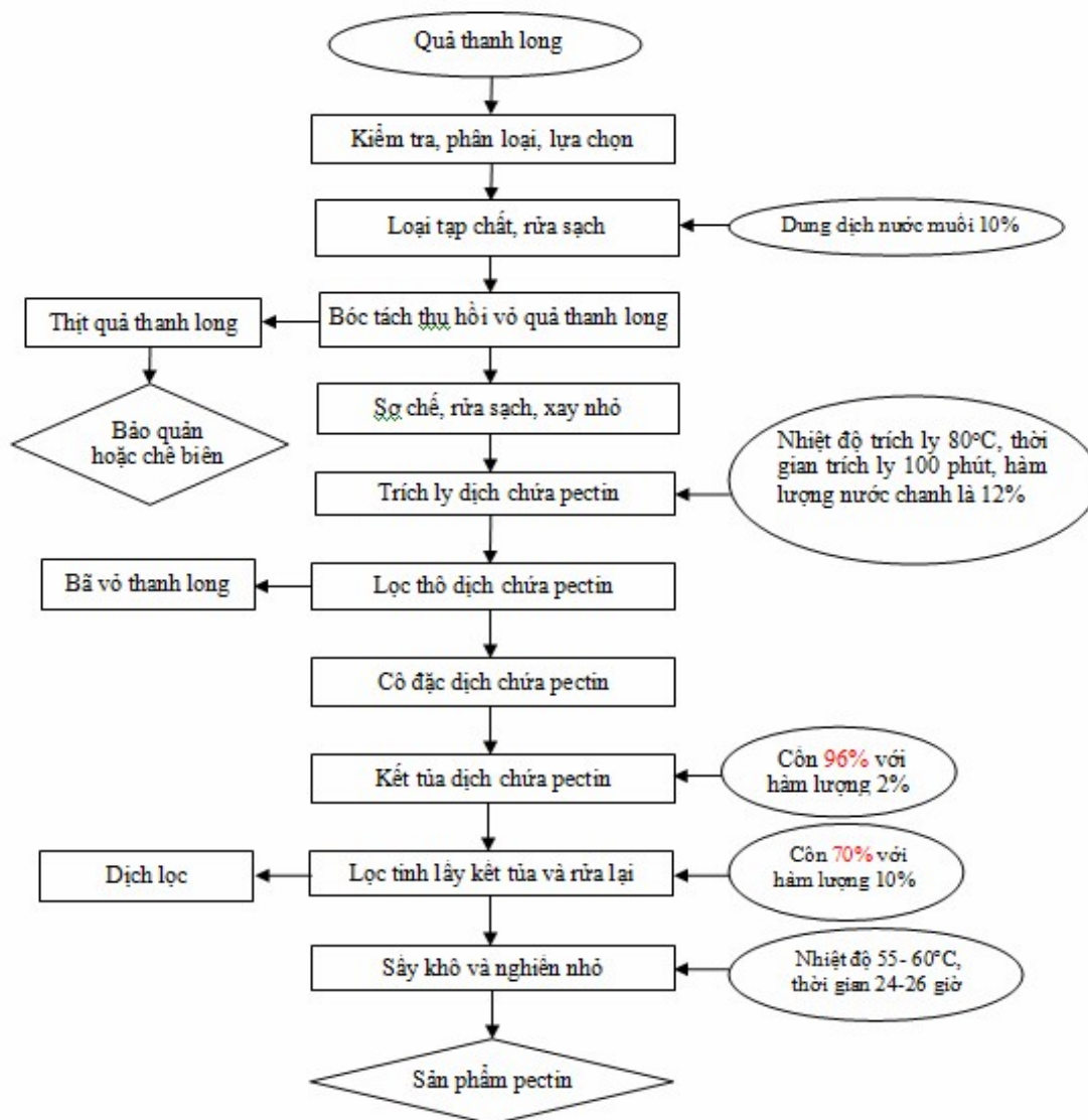
Hình 1. Sơ đồ quy trình khai thác và thu hồi pectin từ vỏ quả thanh long
