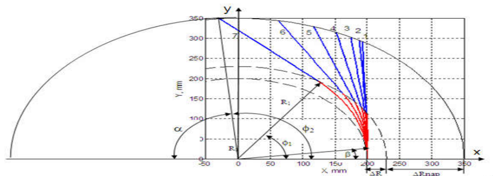
Hình 3. Quỹ đạo khối lạc xét trong hệ quay xOy
