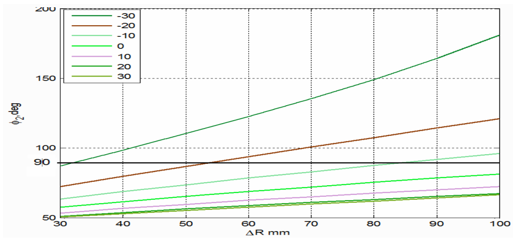
Hình 8. Ảnh hưởng của chiều cao răng tới tới góc tiếp xúc với nắp trống với góc nghiêng răng (độ) khác nhau
