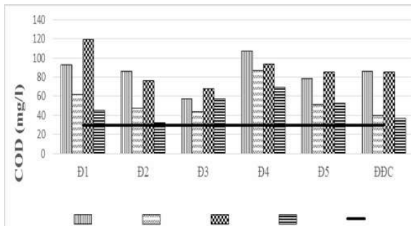
Hình 5. Giá trị thông số COD tại khu vực nghiên cứu
