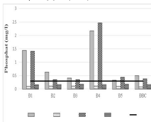
Hình 8. Hàm lượng phosphat tại khu vực nghiên cứu
