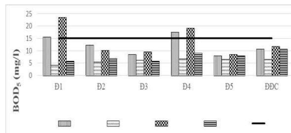
Hình 6. Giá trị thông số BOD 5 tại khu vực nghiên cứu
